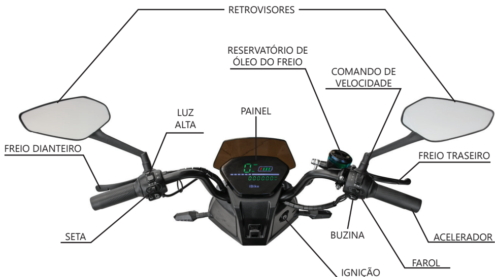
FIGURA 7- COMPONENTES DE CONDUÇÃO
